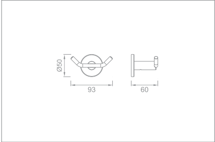
Robe hook Code no.: Q9.110 MP Q9.110 BP
