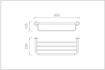
60cm double towel rack Code no.: Q9.012 MP Q9.012 BP
