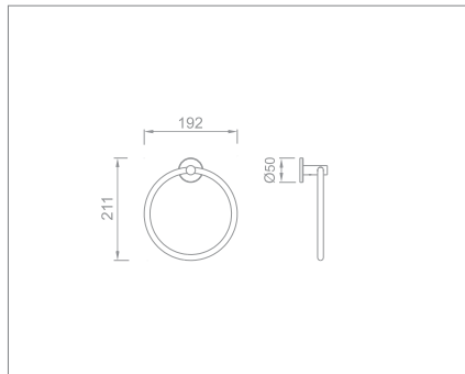
Towel ring Code no.: Q9.004 MP Q9.004 BP
