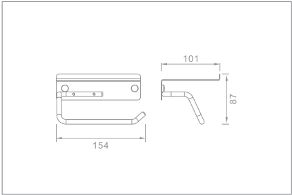
Roll holder with shelf Code no.: Q9.111 MP Q9.111 BP
