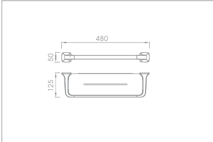
Shelf Code no.: 88003
