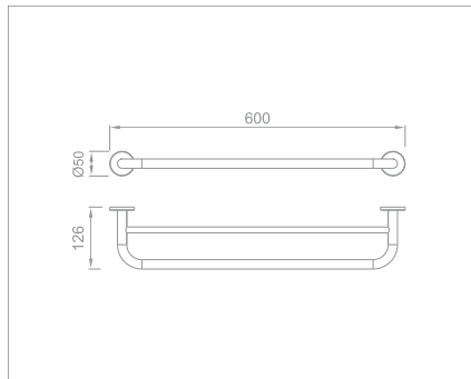
60cm double towel bar Code no.: Q9.002 MP Q9.002 BP
